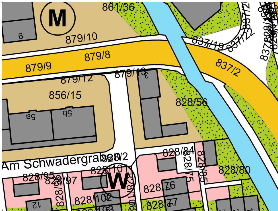
Flächennutzungsplan Bestand
